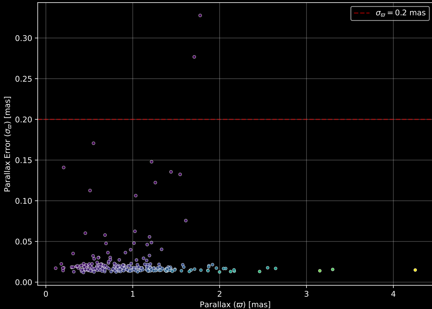
GALAH DR4 Field: [9275] Parallax Quality (n= 278)
