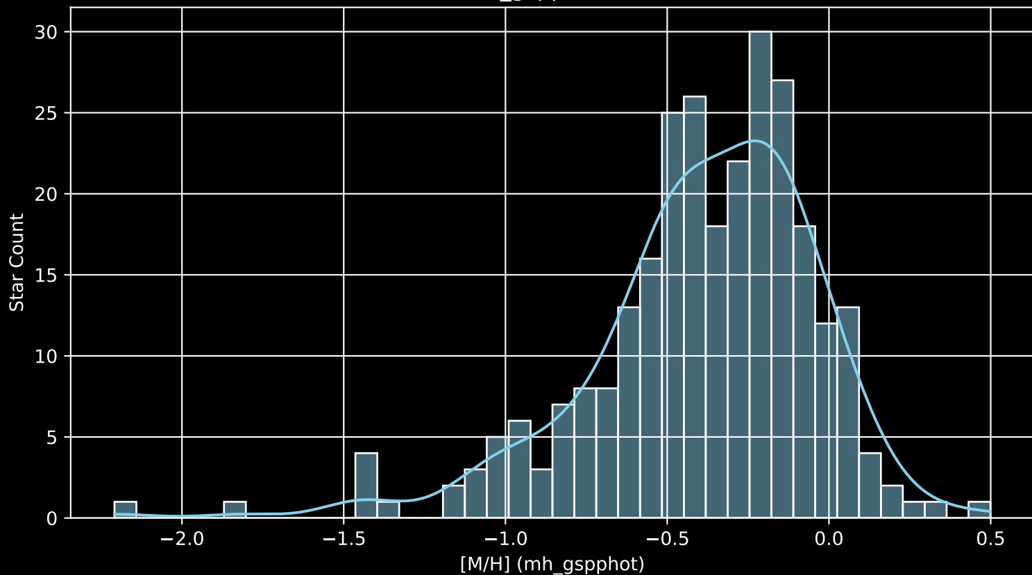
GALAH DR4 Field: [9275] [M/H] (mh_gspphot) (n= 278)
