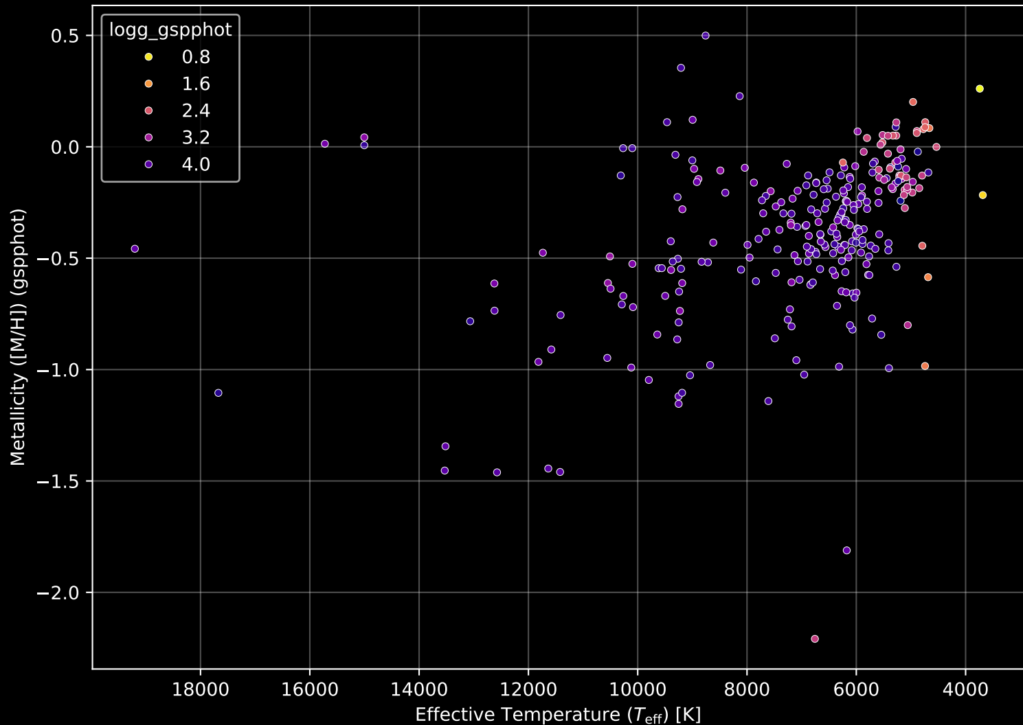
GALAH DR4 Field: [9275] Stellar Population Parameters (n= 278)
