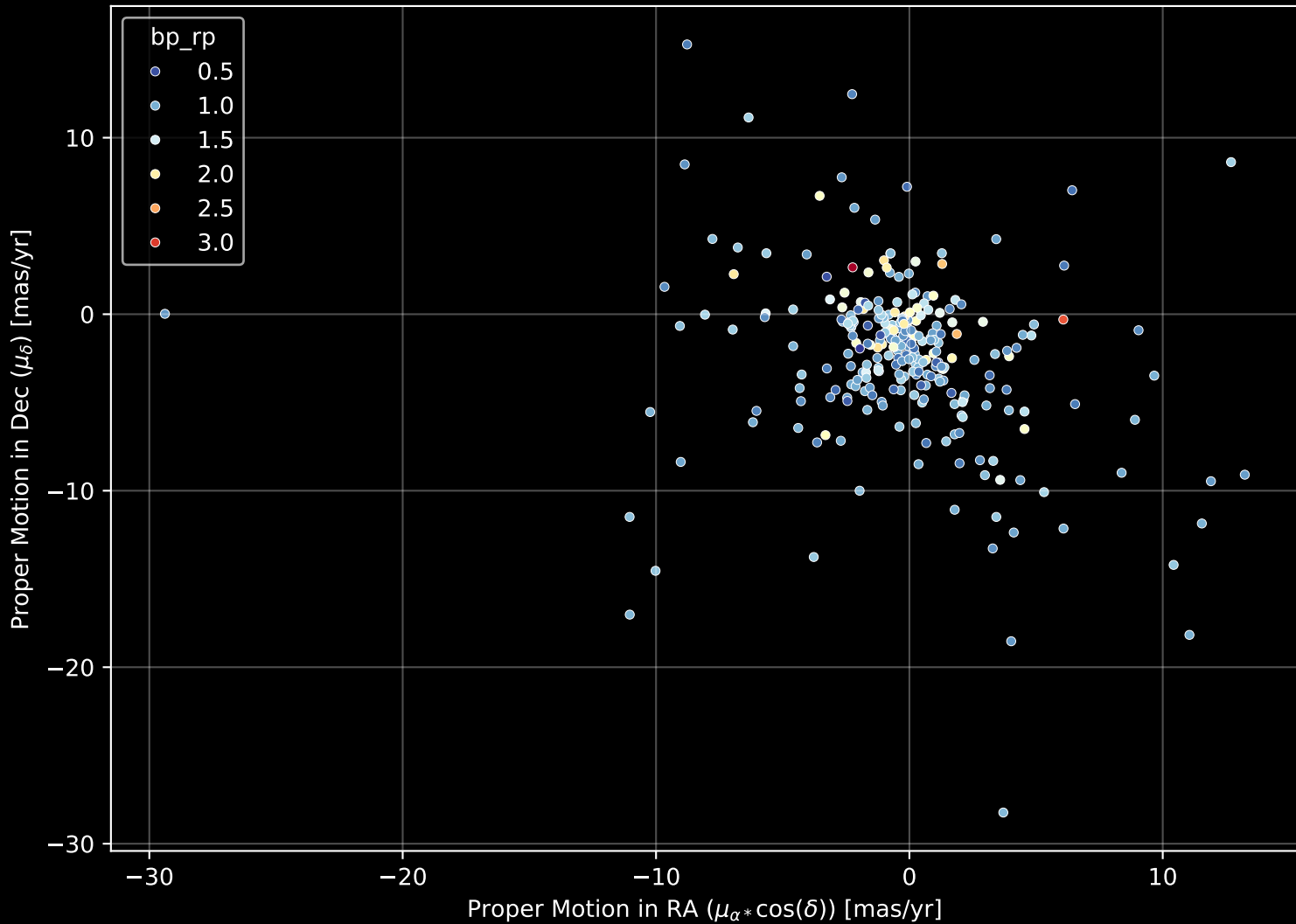
GALAH DR4 Field: [9275] Proper Motion Diagram (n= 278)
