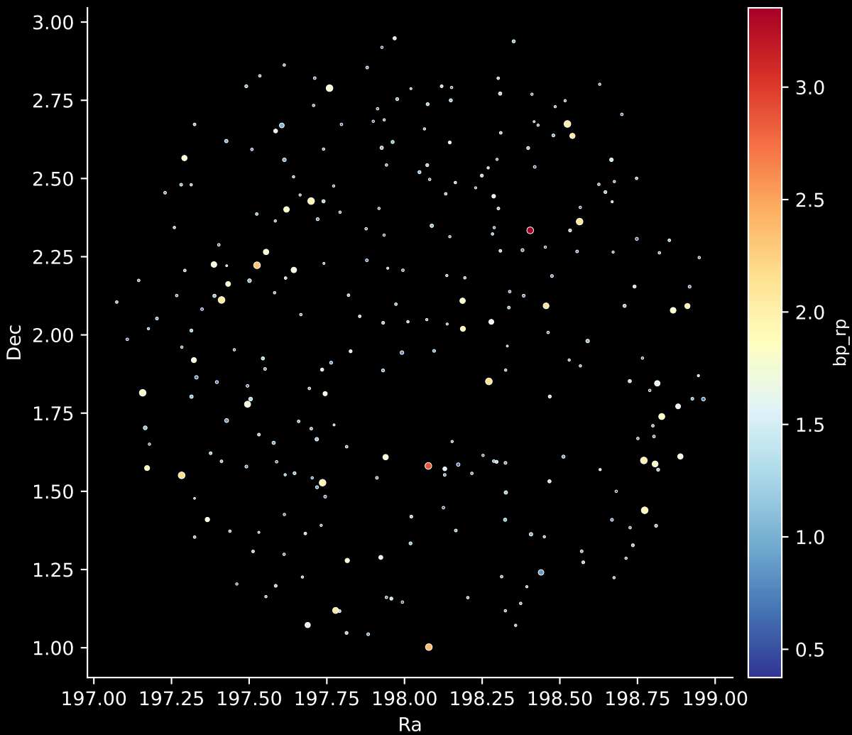
GALAH DR4 Field: [9275] Stars: 278
